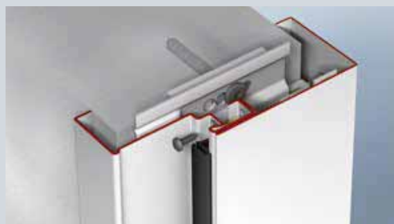
Через канавку для уплотнения привинтить профиль 2 доборной коробки к профилю 1 и затем вставить поверх данного соединения уплотнение двери
