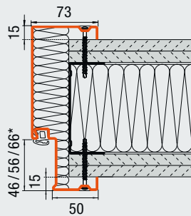
Охватывающая коробка, монтаж на винтовых соединениях (каркасные стены)
