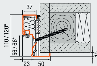
Коробка DryFix с диагональным креплением (деревянные каркасные стены F90 В)
