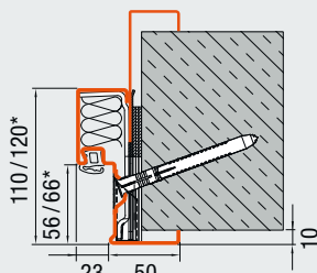
VarioFix Fire (кирпичная кладка/бетон)
